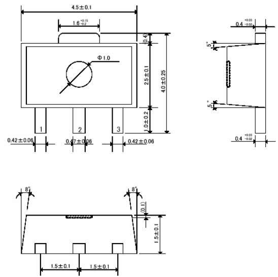
SOT-89
